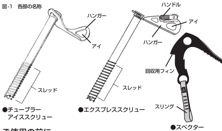
図-1 各部の名称
