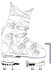
アルパインソールブロック(DIN ISO 9462 適合のアルペンビンディングに対応)
